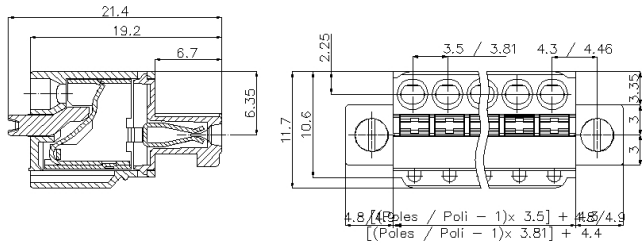
Flange screw M2.5 Flangia a vite M2.5
