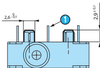
1 Anschluss X2
