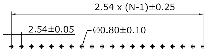
P.C.B LAYOUT
